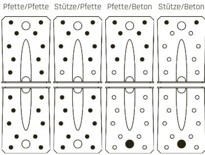
TYP 65/90S 1,5 GREENLINE mit Steg 6503S15
