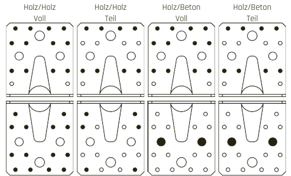
KR Rundloch 135 mm 1101353 / 110135
